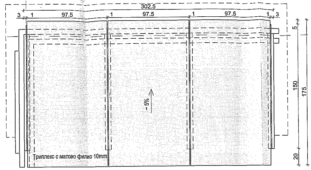
ПЛАН НА ПОКРИВА М 1:20
