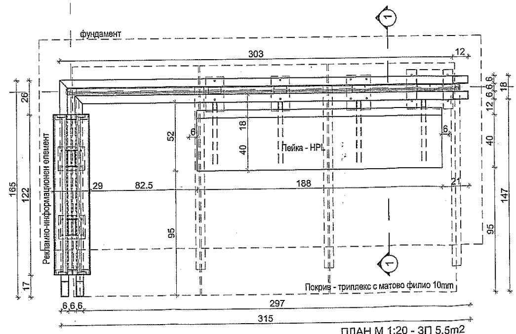
ПЛАН М 1:20 - 3ГП 5.5m2
